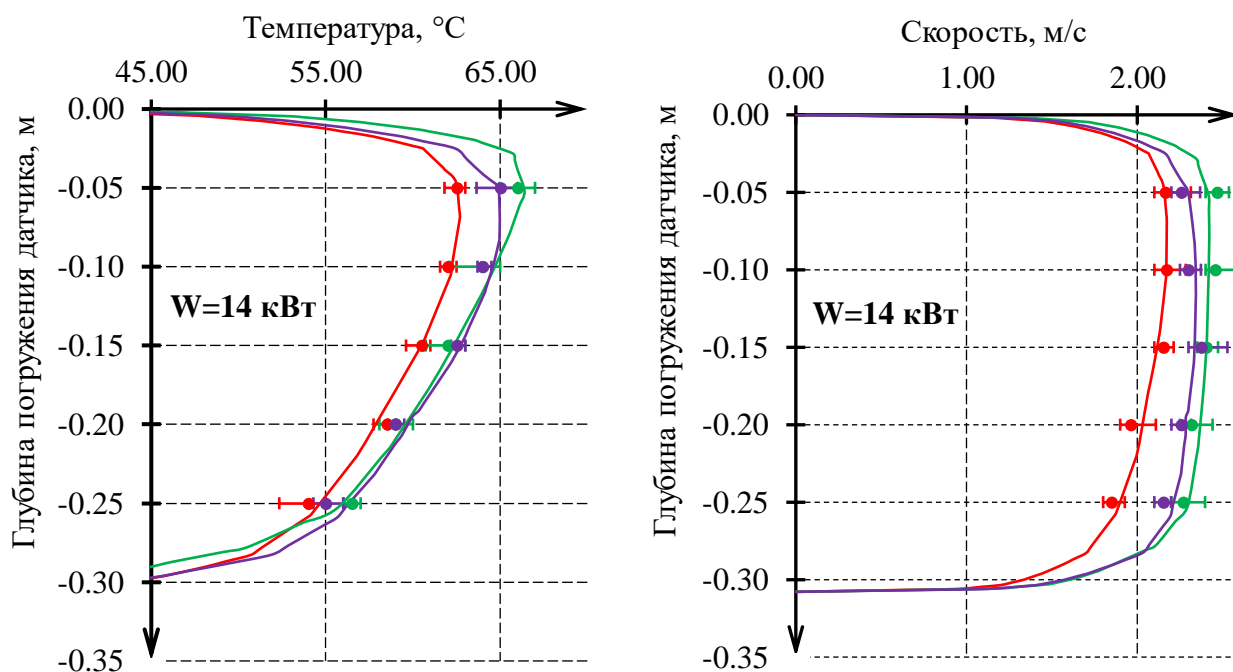
Рисунок 4— Данные натуральных измерений скорости и температуры в сравнении с математической моделью в различных точках сечения 3 при угле наклона – 13 градусов (сиреневый – левая ось, зеленый – центральная ось, красный – правая ось измерения)
