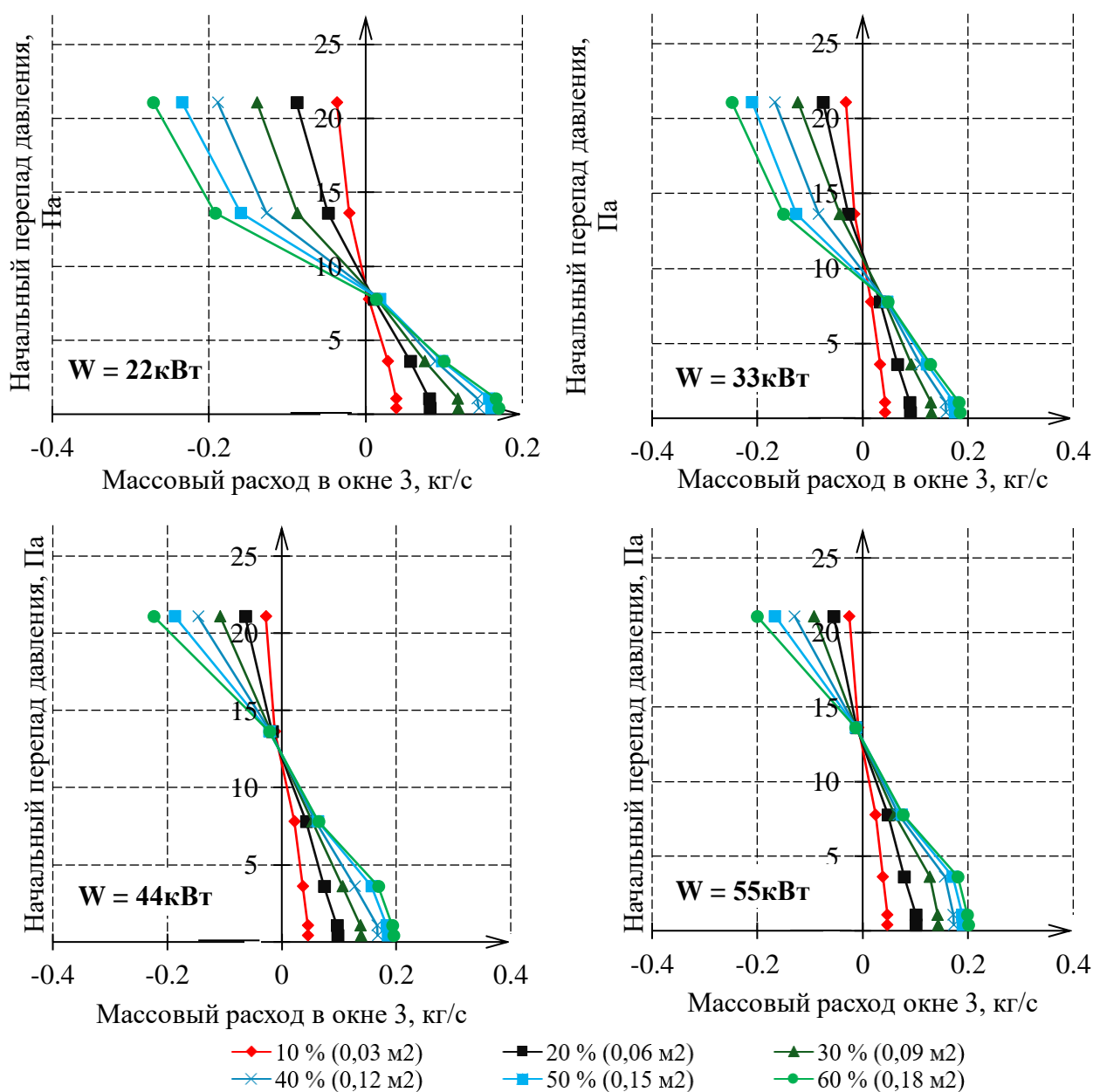
Рисунок 5 — Изменение массового расхода воздуха в отверстии 3 от начальной скорости воздушного потока (перепада давления) при различной степени его открытия
